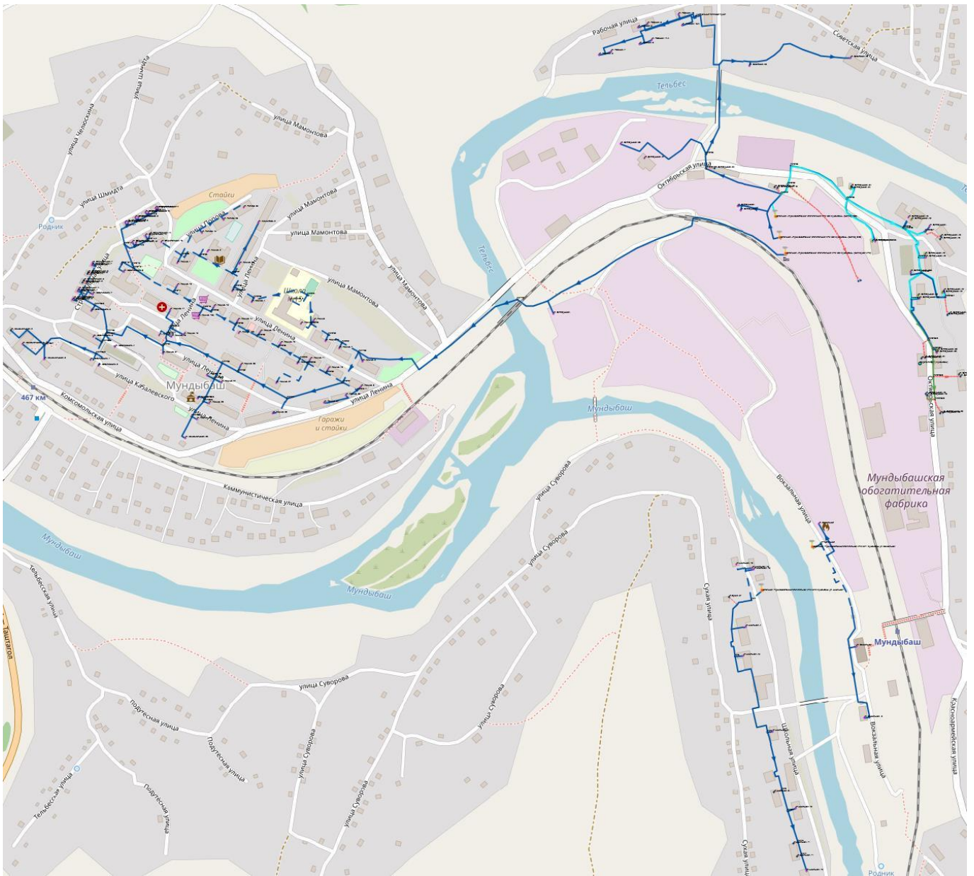
Рис. 13. Визуальное отображение структуры тепловых сетей от источников тепловой энергии п.г.т. Мундыбаш
