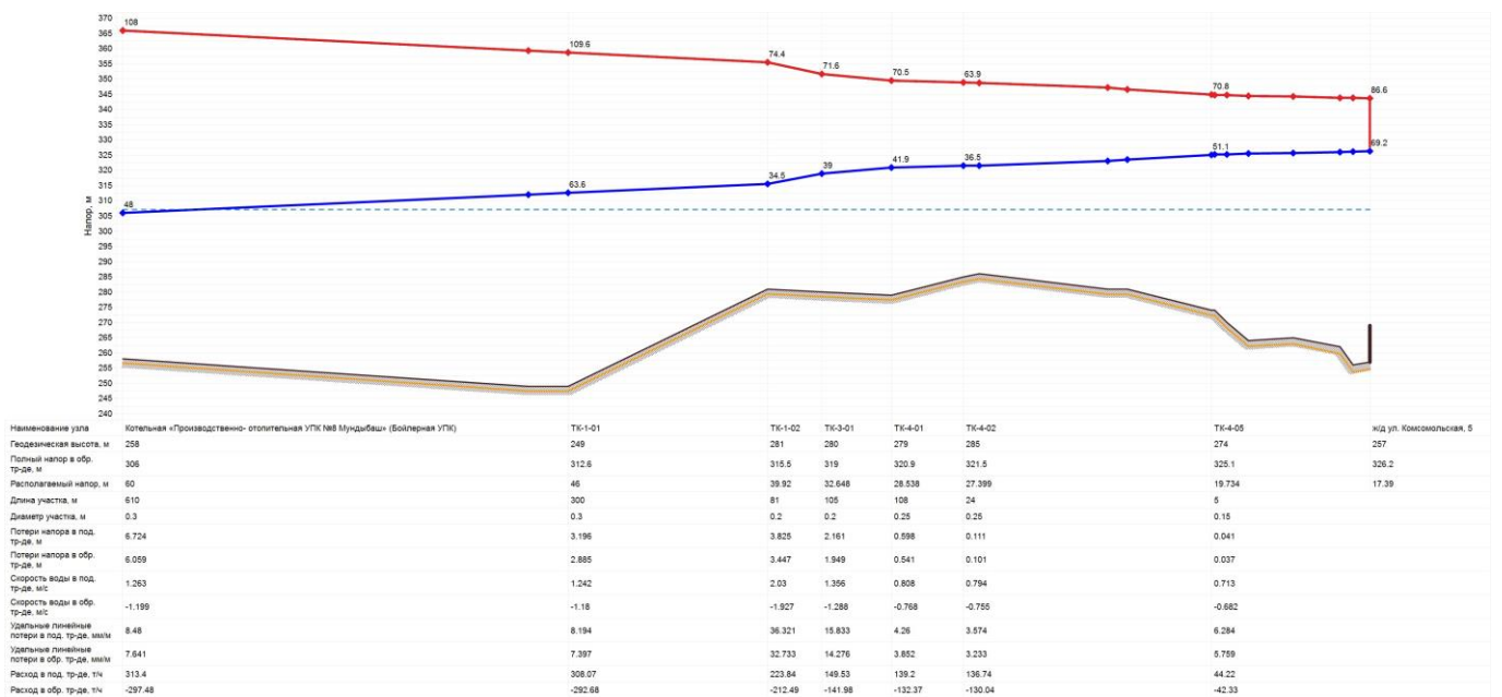
Рис. 12. Пьезометрический график
