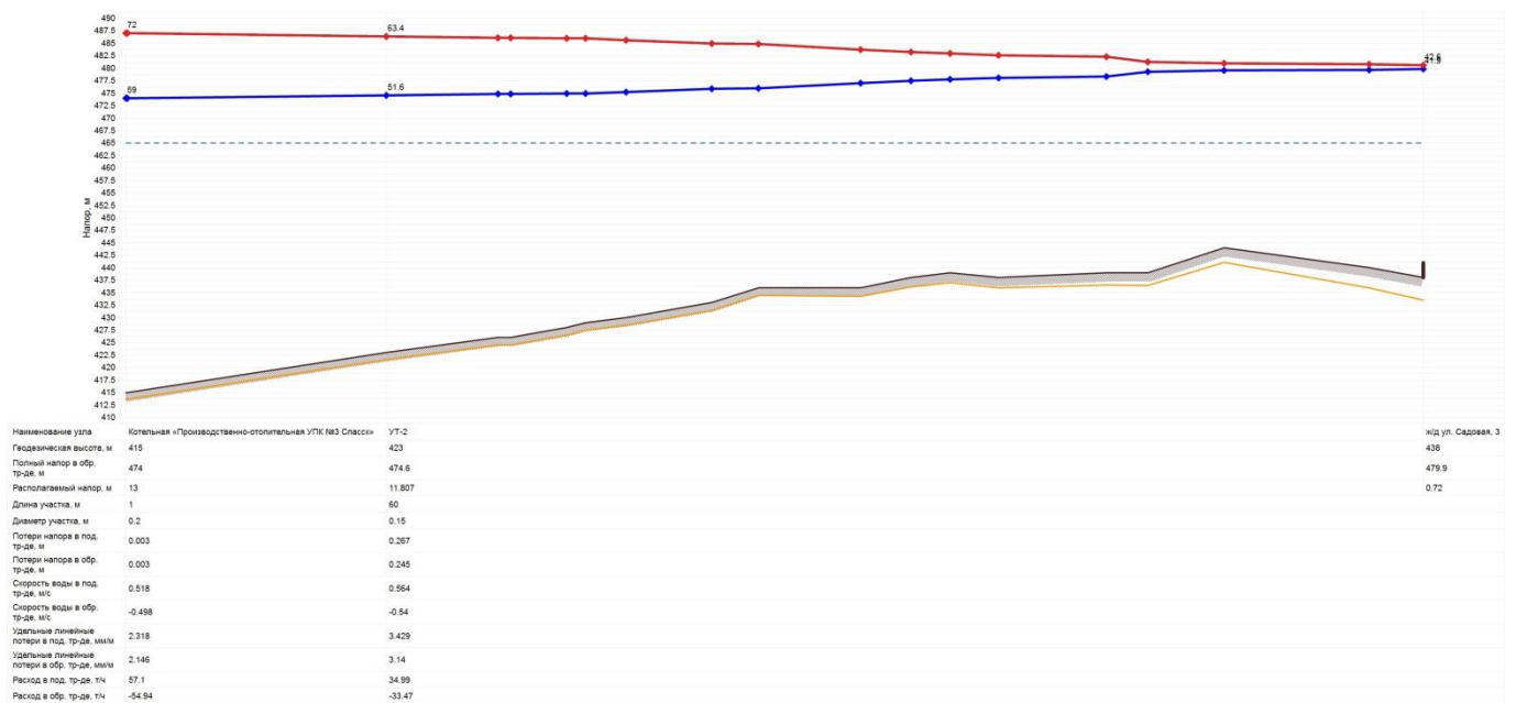
Рис. 12. Пьезометрический график
