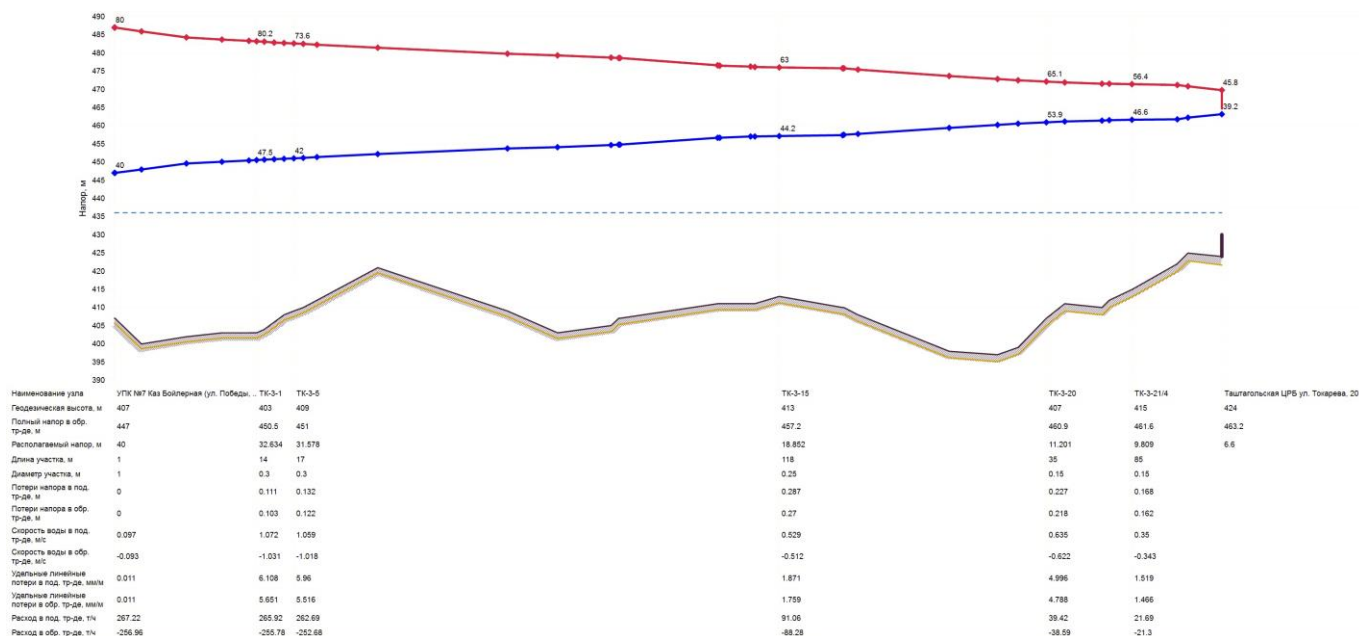
Рис. 12. Пьезометрический график
