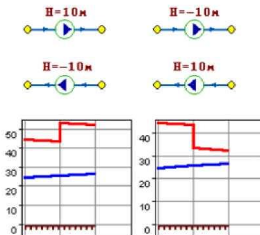
Рис. 7. Пьезометрические графики
