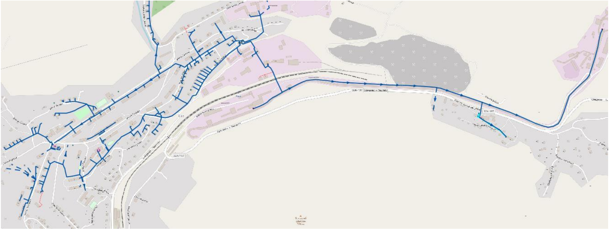
Рис. 13. Визуальное отображение структуры тепловых сетей от источников тепловой энергии п.г.т. Каз
